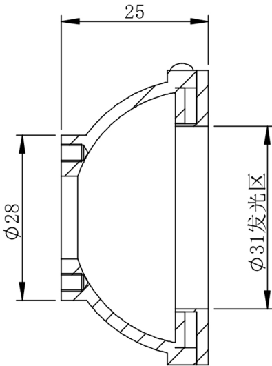
剖面 C-C
