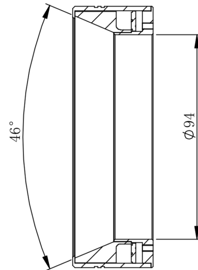
剖面 F-F
